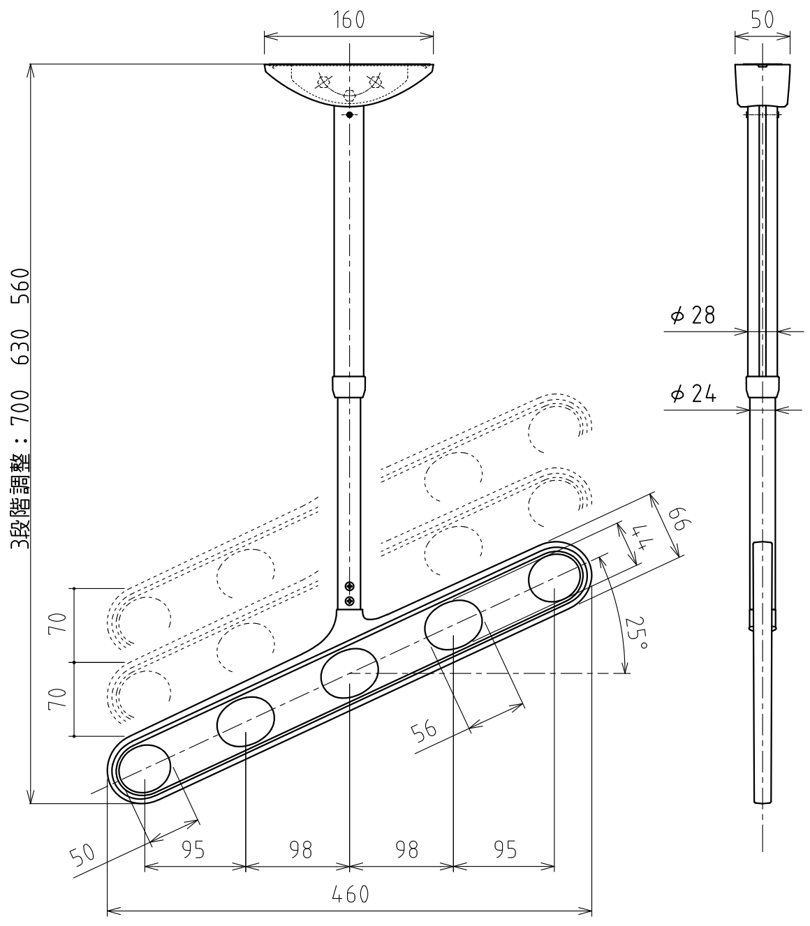
ホスクリーンZAN-0650型 製品図
