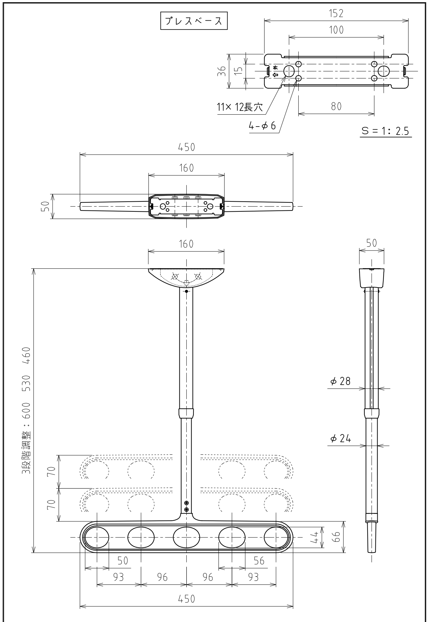
ホスクリーンZA-0645型 製品図
