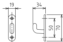
④ 操作棒かけフック (S=1/3)
