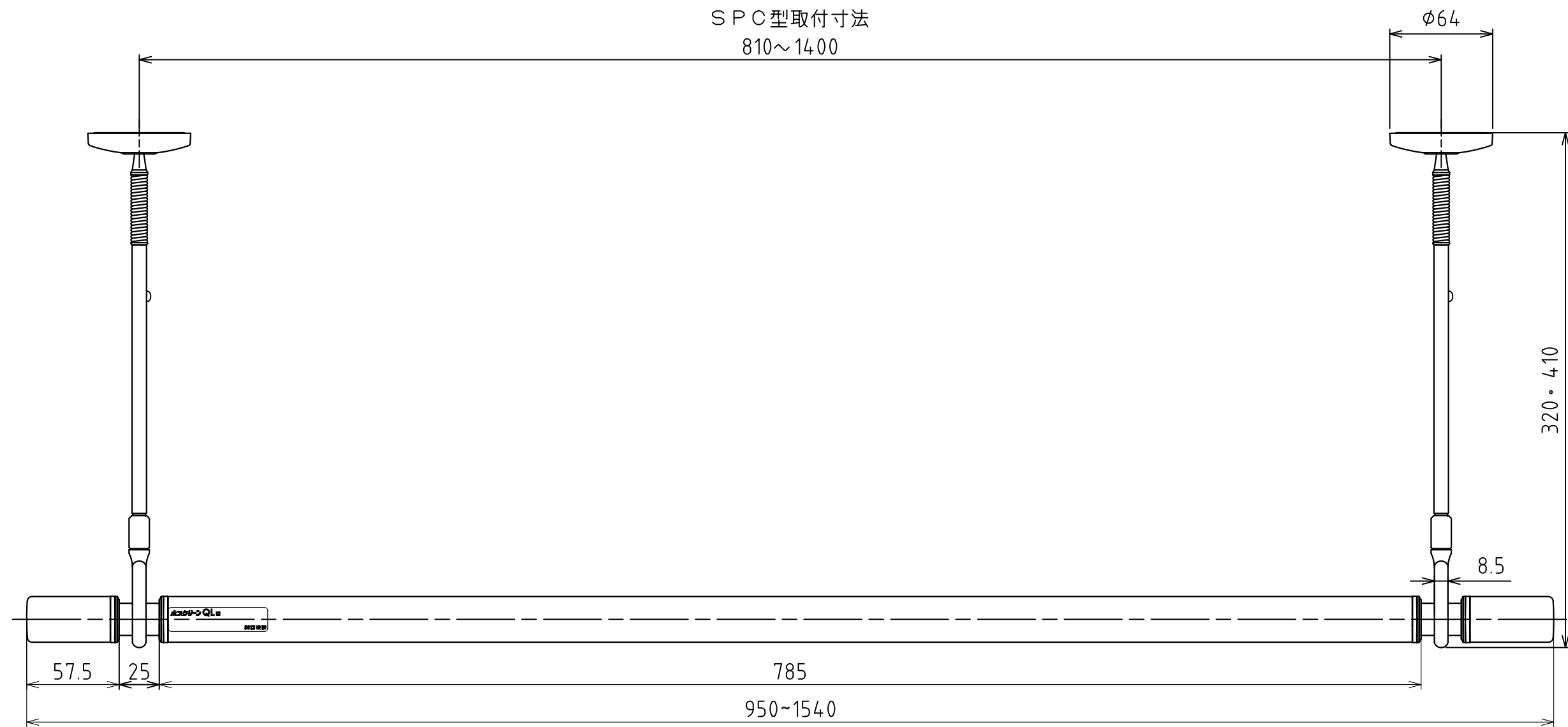
[ポール掛けフック]
