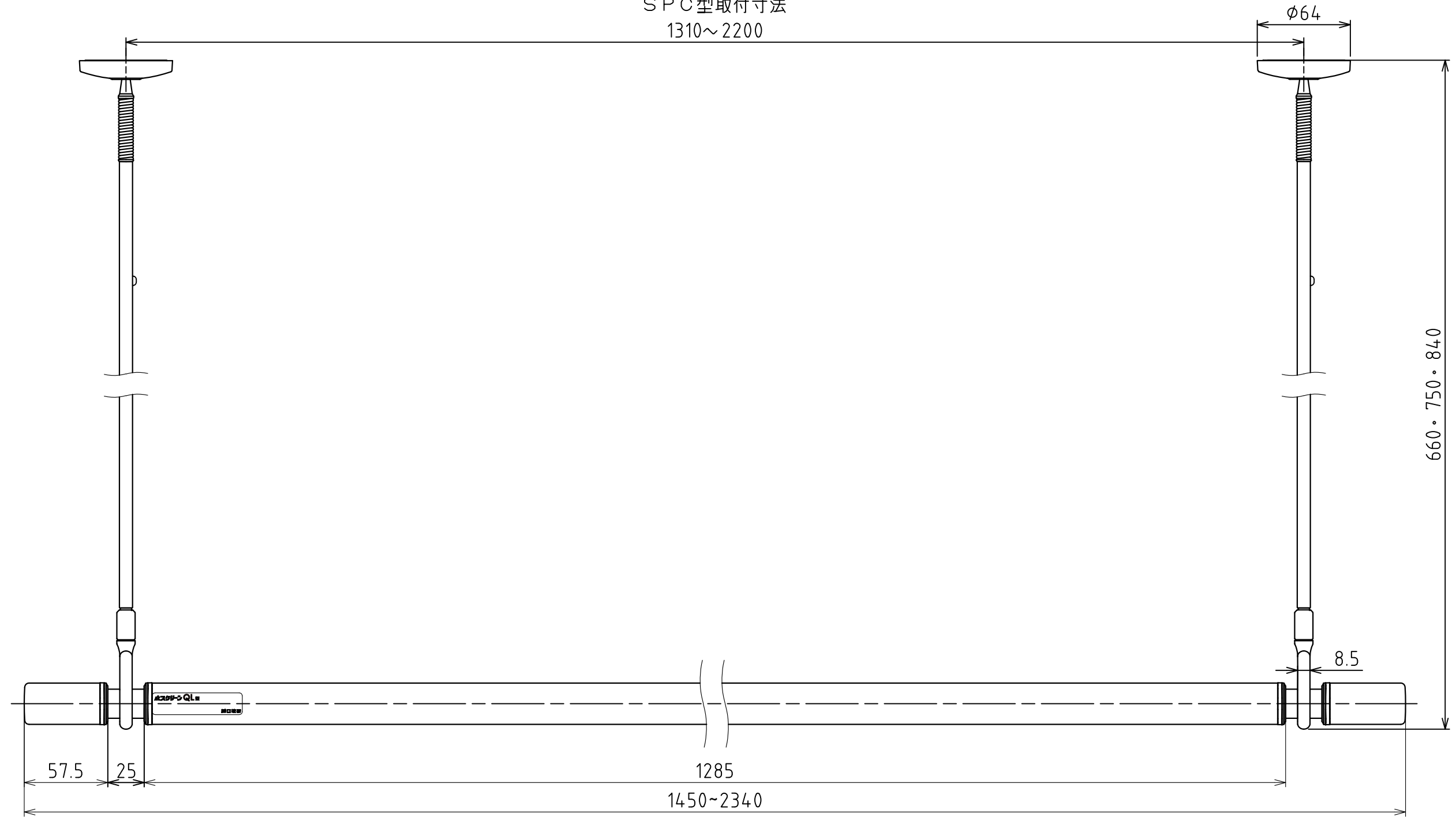
〔ポール掛けフック〕
