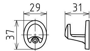
〔SPC型取付ネジ〕 TPネジ φ4×50
