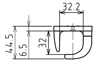
[竿立てホルダー]
