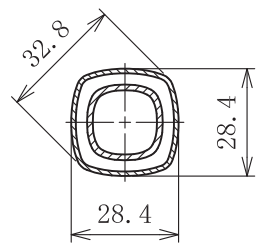
A-A断面図
