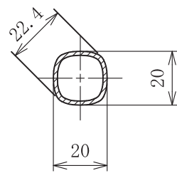
B-B断面図
