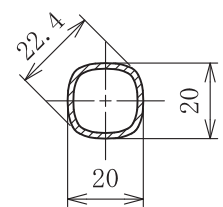
B-B断面図
