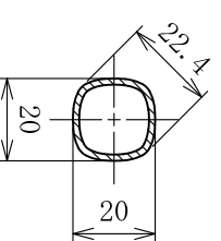
B-B断面図
