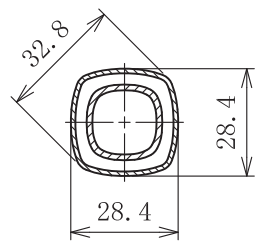
A-A断面図
