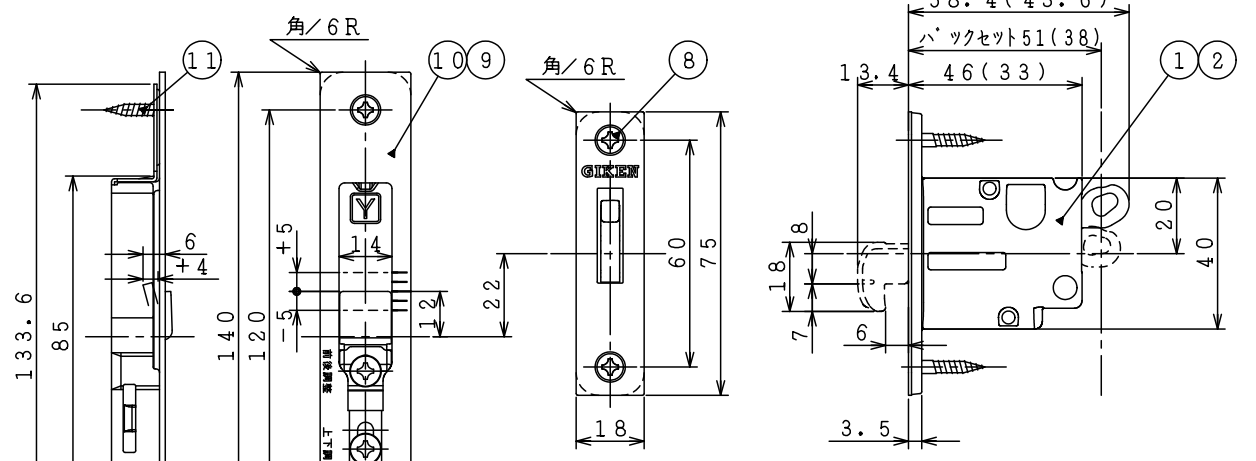
図はDY151引戸錠。 ( )内の数字はDY138引戸錠の数値です。
