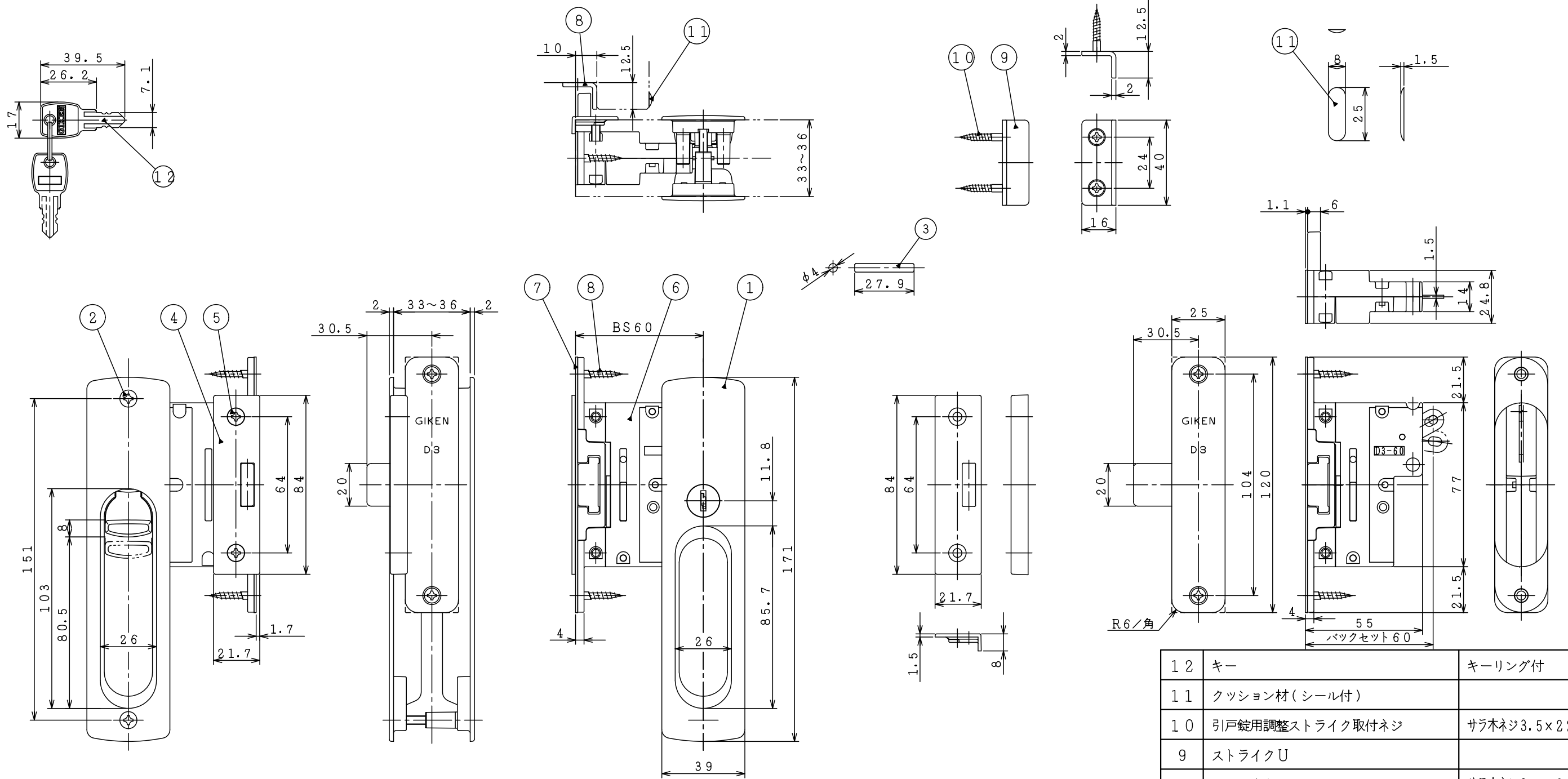
本図はR(右勝手)仕様を表す。
