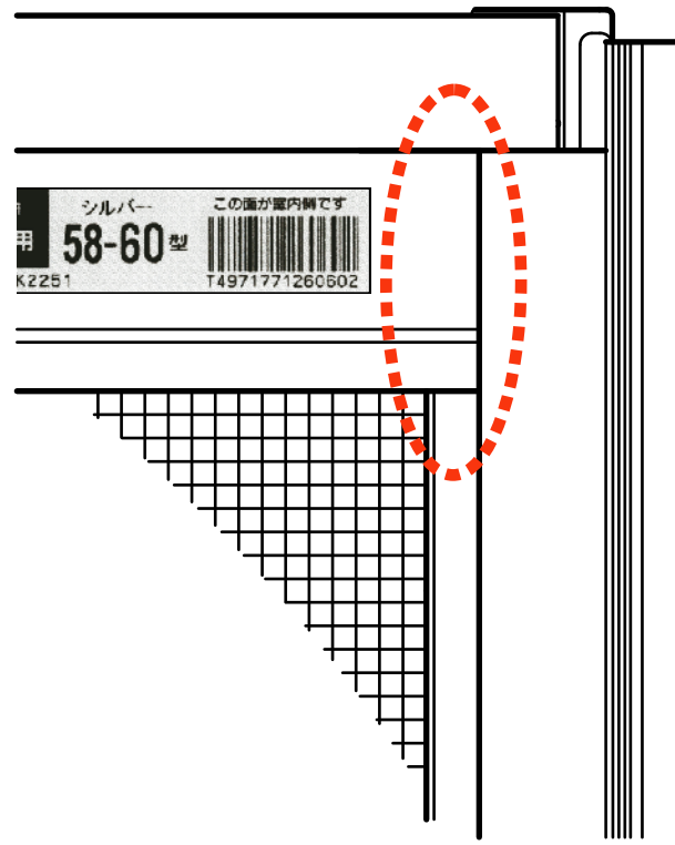
タテとヨコは直角カットしたジョイント
