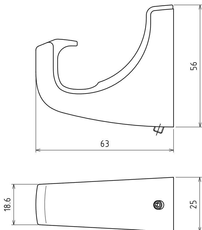
〔本体〕
