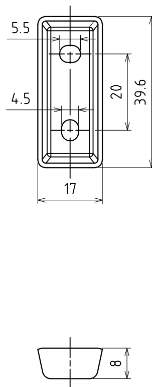
〔取付座〕
