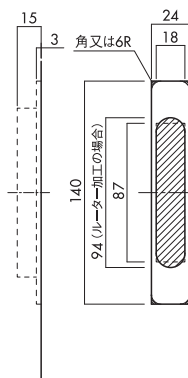
扉側加工(引手のみ)
