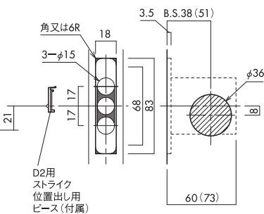
扉側加工 (D2セパレートタイプ引戸錠用鎌錠+本体)
