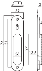
3A/4A(室外)
