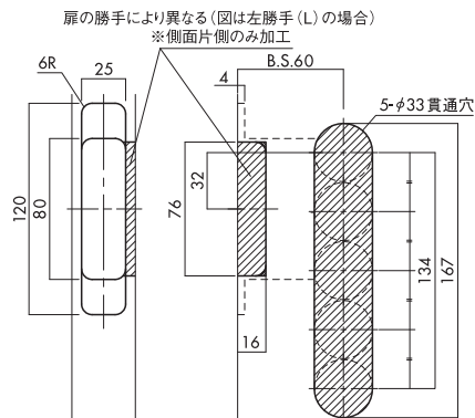
扉側加工(D3アウトセット引戸用錠+本体)
