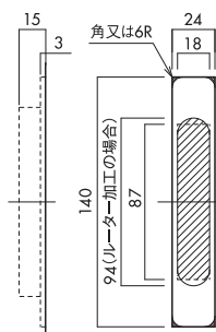
枠側加工 (YK/Y6調整ストライク)
