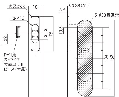
扉側加工(DY1引手一体型引戸錠用鎌錠+本体)
