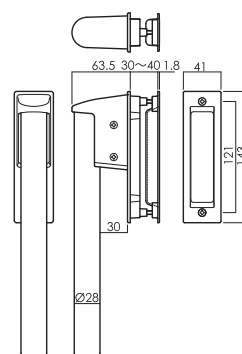
BH-K1G(片面バー引手タイプ)
