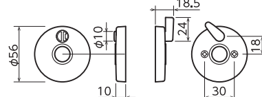
丸座内締錠 / 表示錠
