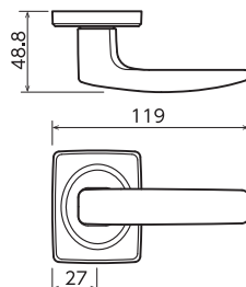
戸襖用ハンドル
