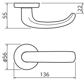
ハンドル No.43
