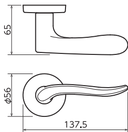
ハンドル No.32
