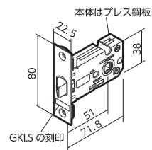
LSミニケース錠
