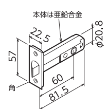
戸襖用ラッチ本体 BS-60
