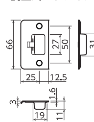
NS-25 調整式ストライク
