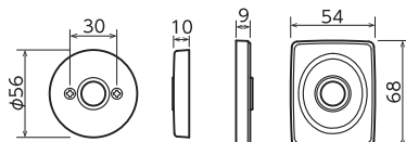
丸座戸襖錠
