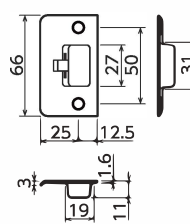
NS-25 調整式ストライク
