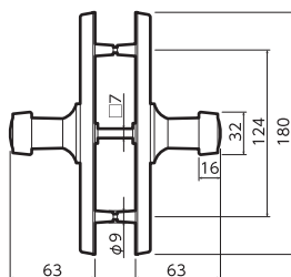
長座 握り玉錠
