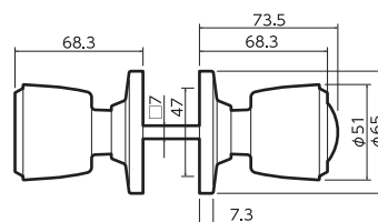
内鍵付 (非常開錠機構付)
