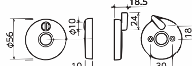
丸座内締錠 / 表示錠
