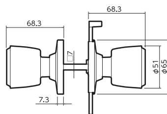
内鍵付 (非常開錠機構付)
