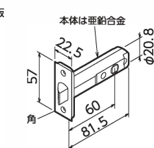
戸襖用ラッチ本体 BS-60
