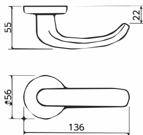
ハンドル No. 43
