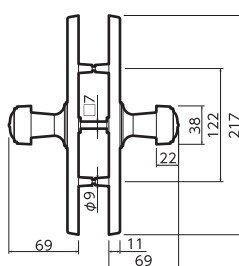
長座 握り玉錠
