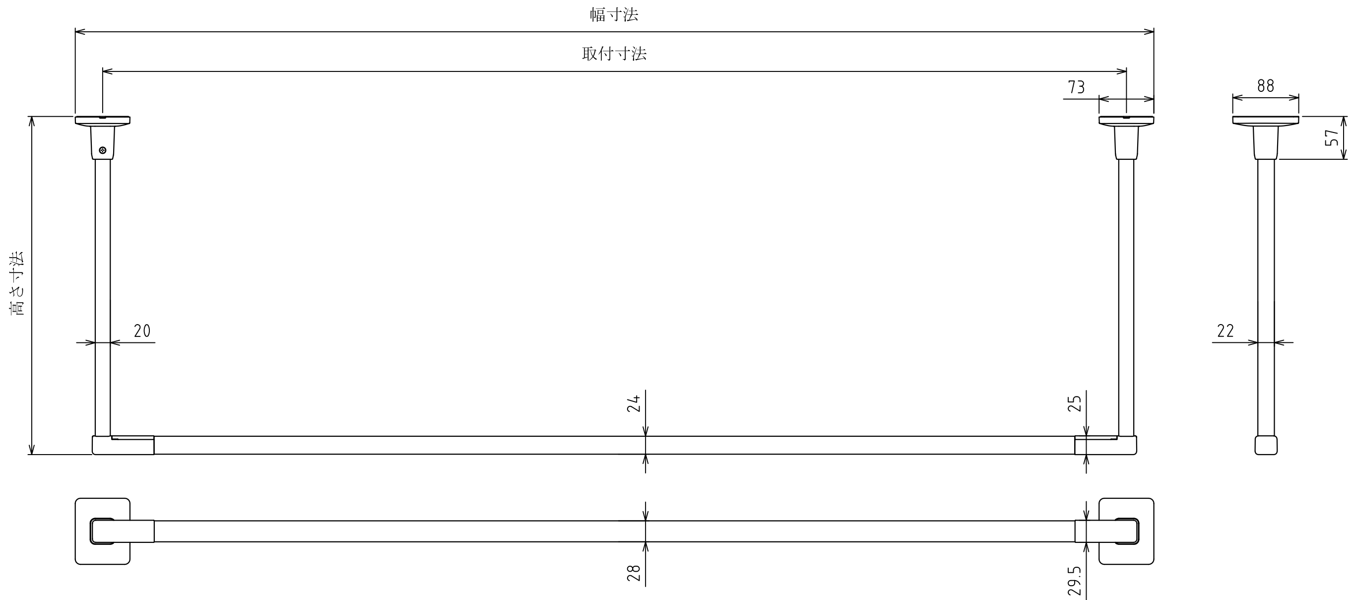
■寸法表
