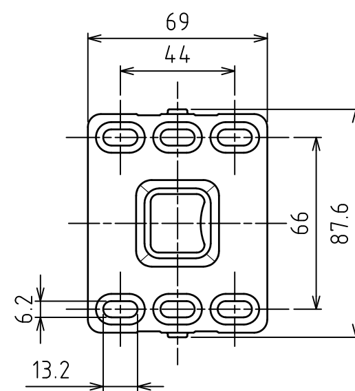
■ベース寸法
