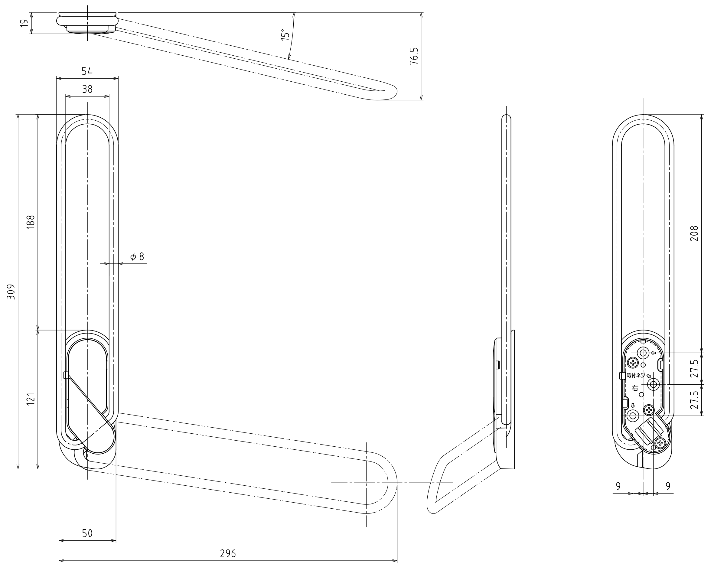
ホスクリーンMDL型 製品図
